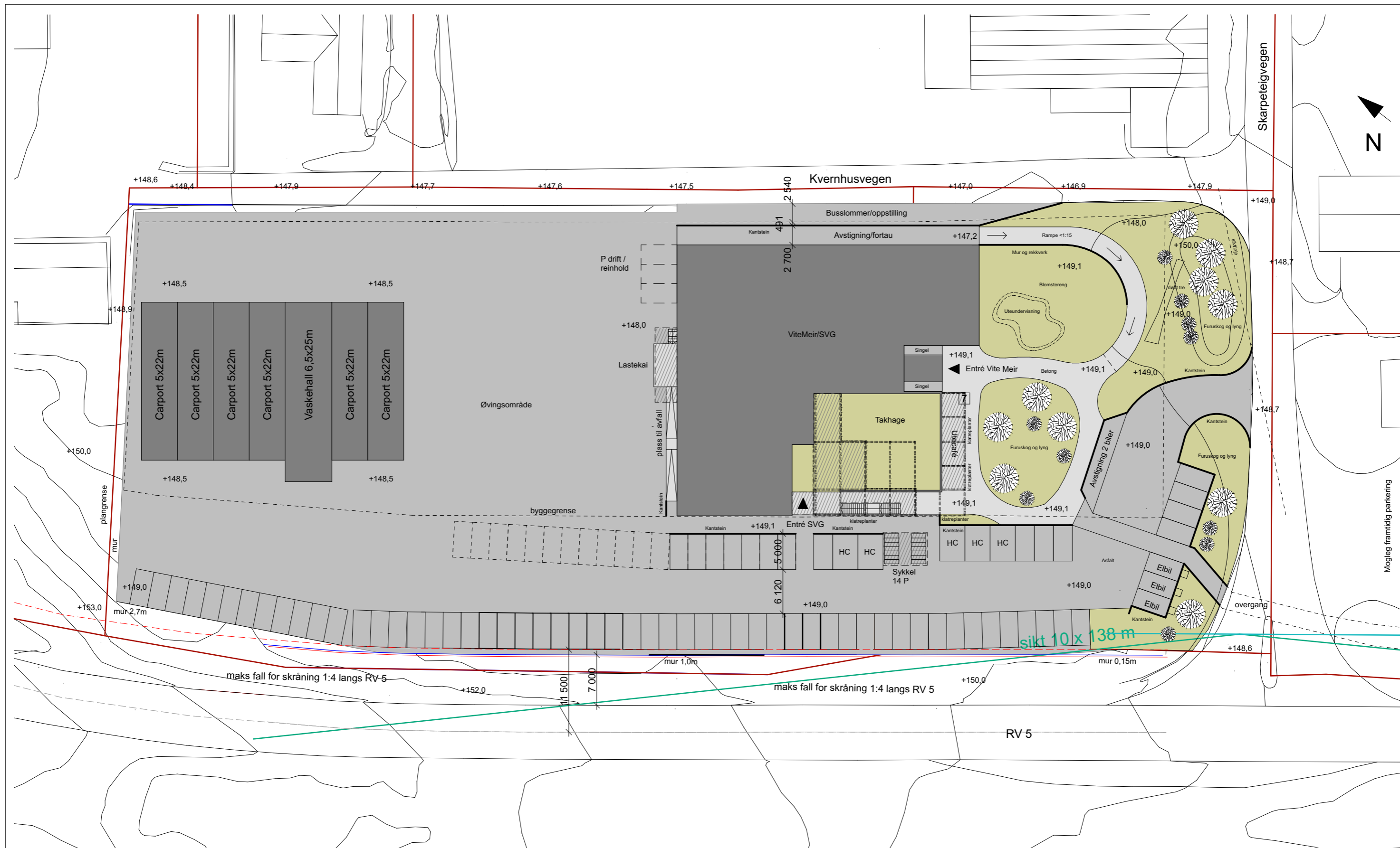
1:500 Situasjonsplan
