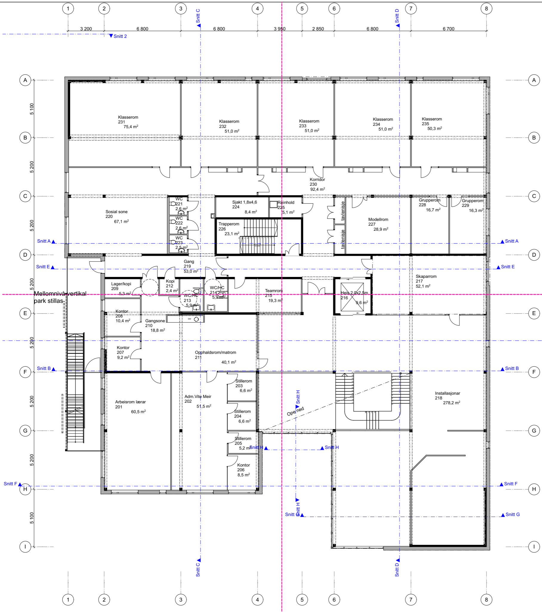
1:200 Plan 2. etasje
