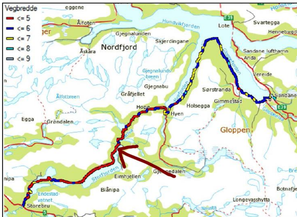
Figur 3.2: Registrert vegbreidde langs fv. 615 (NVDB)
