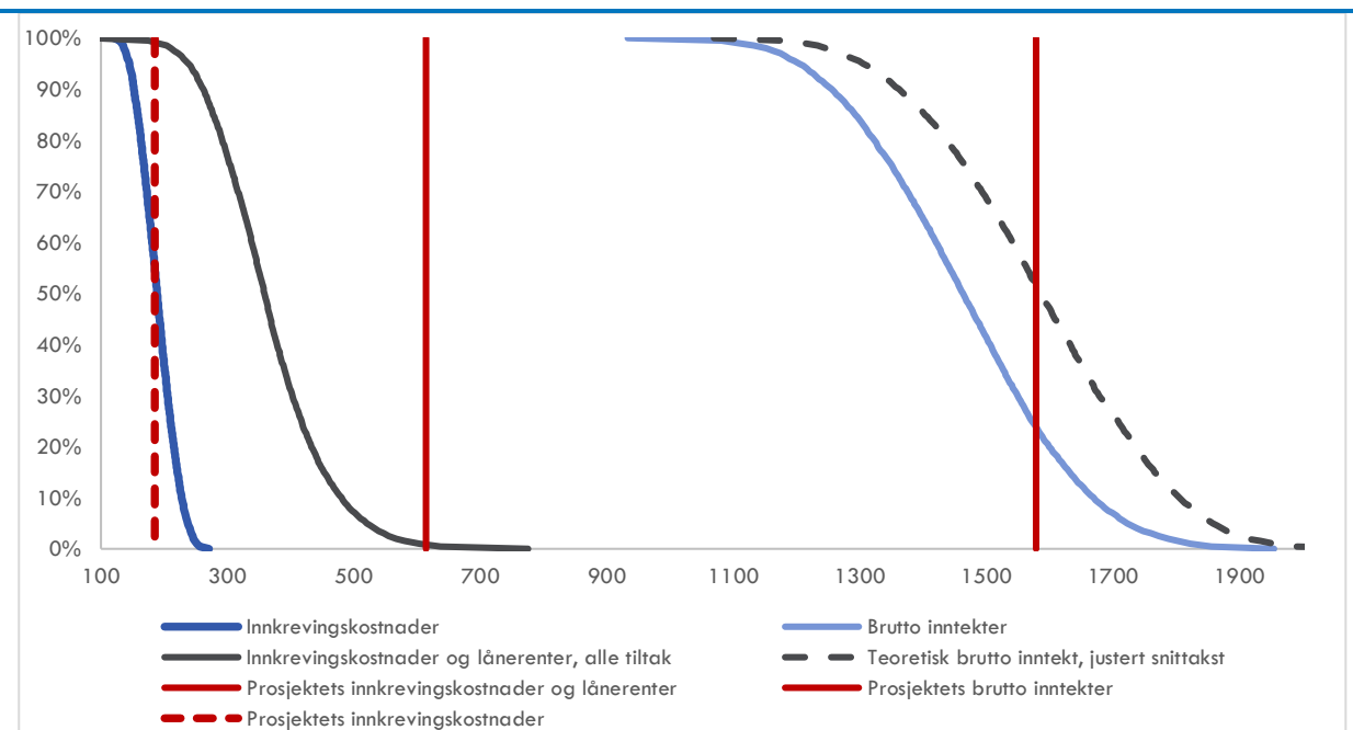
Figur 6-4: S-kurve hovedresultater ved nytt bompengeanlegg, millioner 2020-kroner
