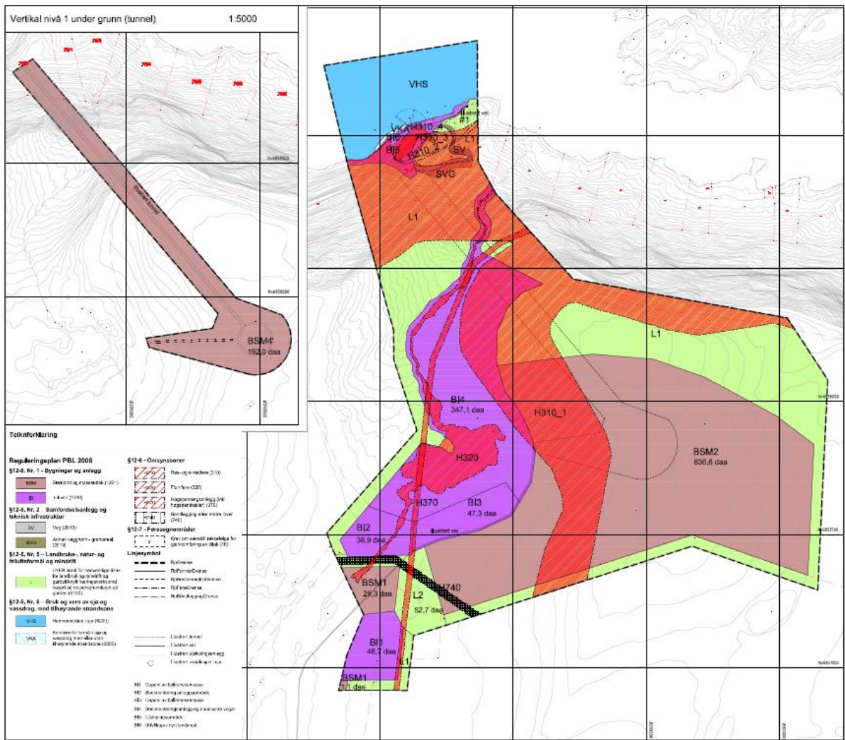
Figur 1-1. Foreløpig forslag til revidert reguleringsplan for Aksla
