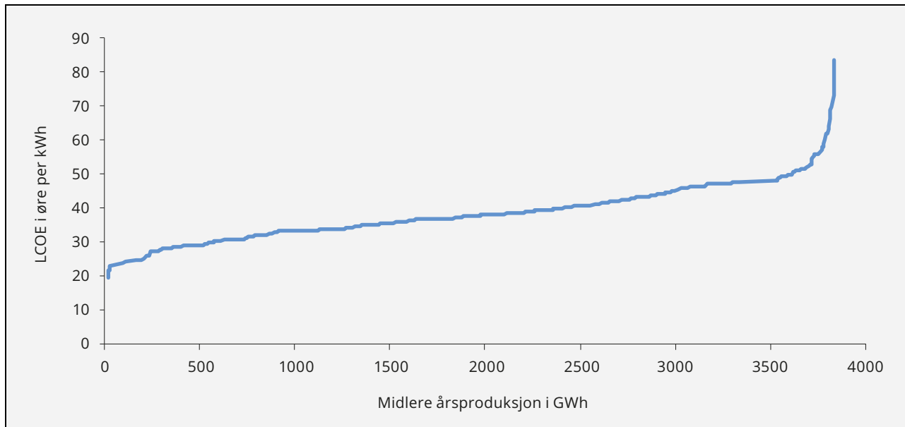
Figur 3.17 Anslag for LCOE for konsesjonsgitte vannkraftverk som ikke er under bygging. Faste 2018-øre
