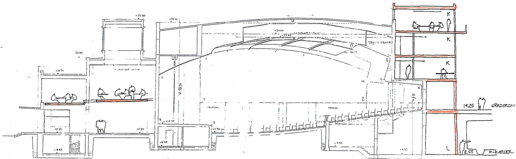
FJØSANGERVEIEN 28 - SNITT - 1:200 - 14.5.08
