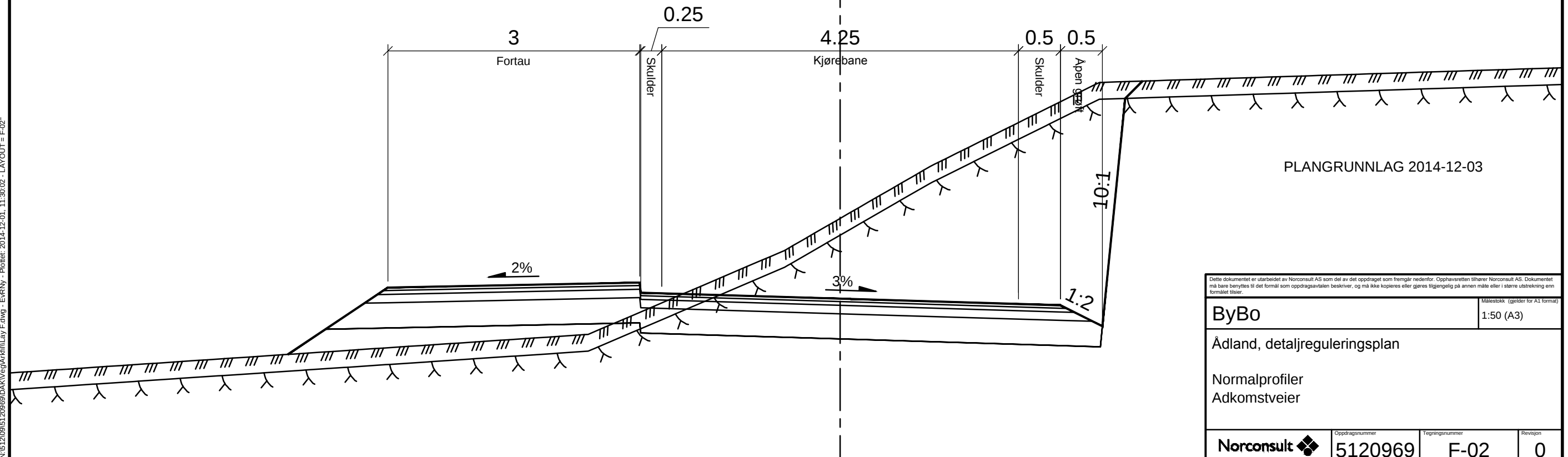
Normalprofil, SKV2b Veglinje 30000 (pr. 200) 1:50
