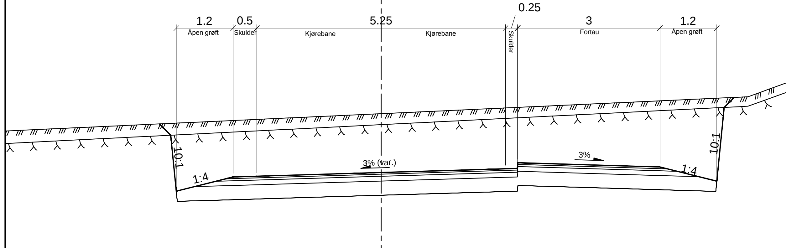
Normalprofil, SKV2 Veglinje 20000 (pr. 0-85) 1:50
