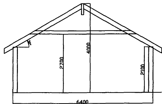
TVERRSNITT
