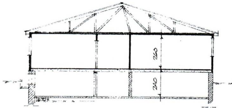
Snittegning.
