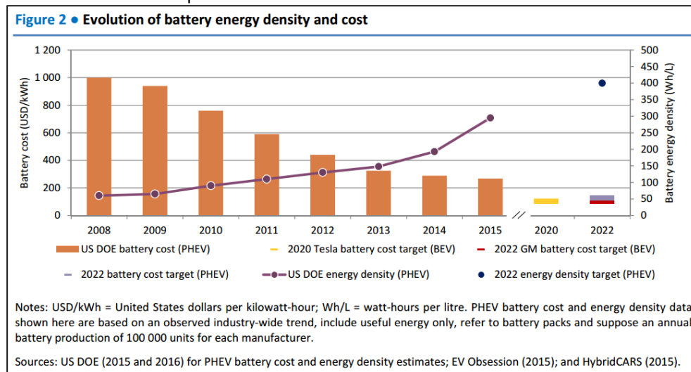
Figur 6: Utvikling av energitettleik og kostnadar for batteri (kjelde: IEA 2016)
