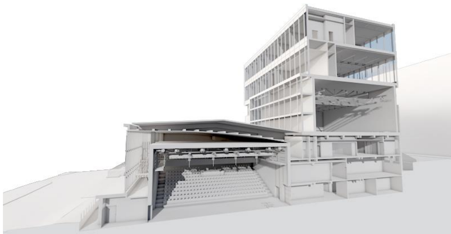
Figur C.5.1 Snitt gjennom hovedscene i plan 0 og monteringsstudio i plan 3-5.
