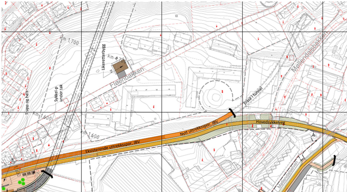
Utklipp fra illustrasjonsplan som viser gang- og sykkelveg fra holdeplass til Kronstad-tunnelen(Sweco)
