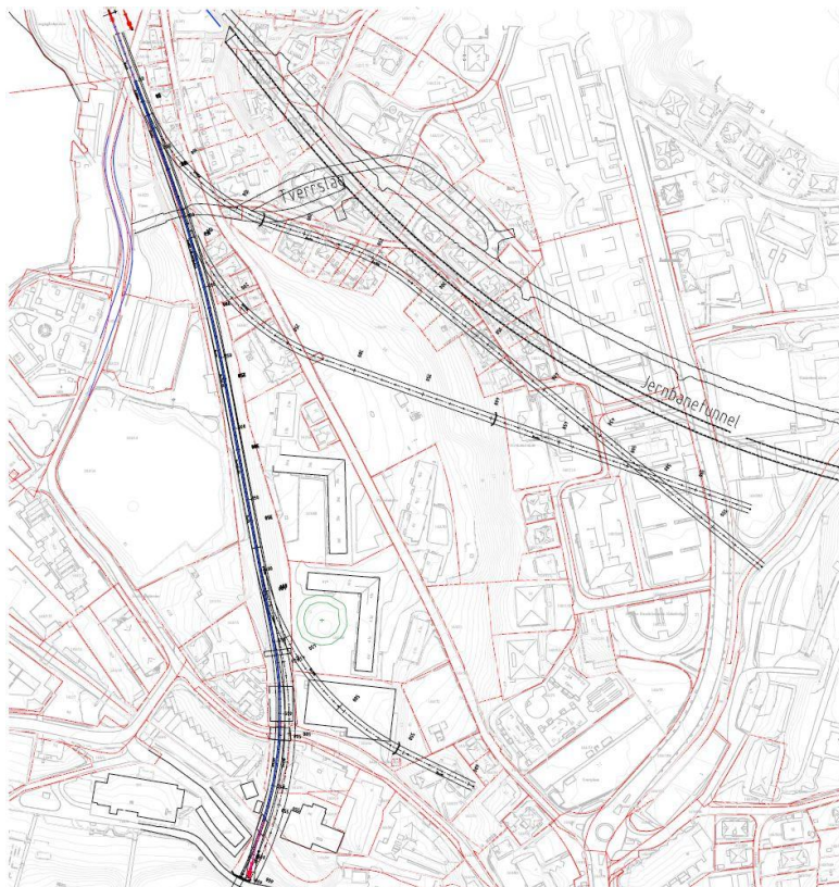
Vurderte traséer for uttrekkspor i Fløen/Møllendal(Sweco).
