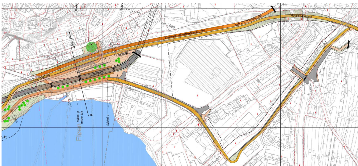
Utklipp fra illustrasjonsplan som viser gang- og sykkelveg fra holdeplass til Kronstad-tunnelen(Sweco)
