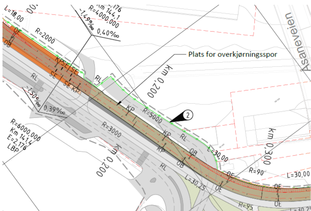
Figur 2: Plassering av overkjøringsspor ved Lungegårdskaien holdeplass
