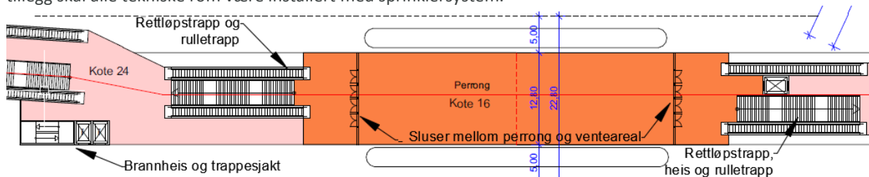
Figur 29 – Prinsipløsning for utforming av holdeplass på kote +16 med tilhørende brannsluser mellom perrong og trappe-ventearealer
