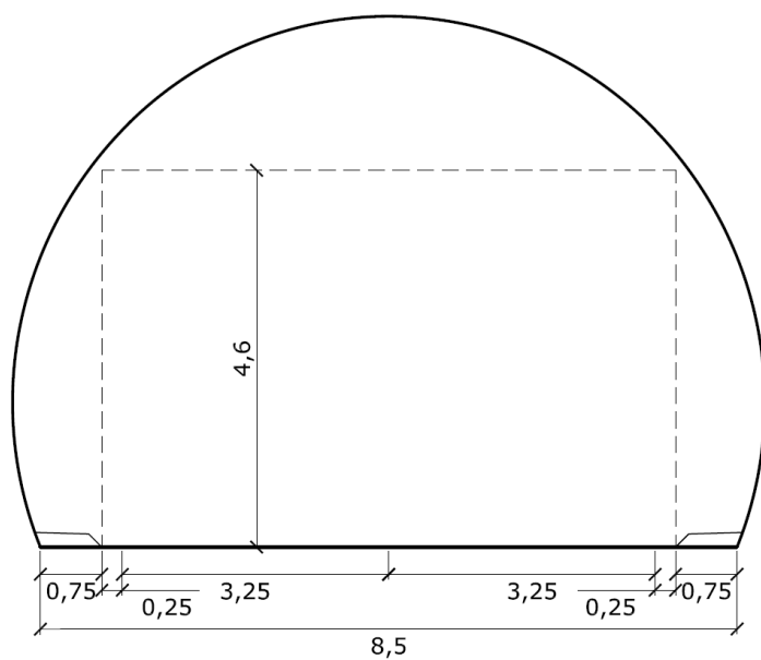
Figur V1.12 Tunnelprofil T8,5 (mål i m).
