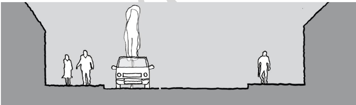
Figur B.6: Gate med langsgående parkering og to kjørefelt. Minste bredde mellom parkerte kjøretøy og kantstein bør være 4,5 m
