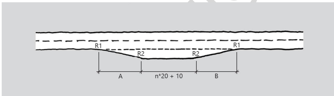
Figur D.37: Busslomme uten trafikkdeler, n angir hvor mange busser som forventes å stoppe samtidig (mål i m)
