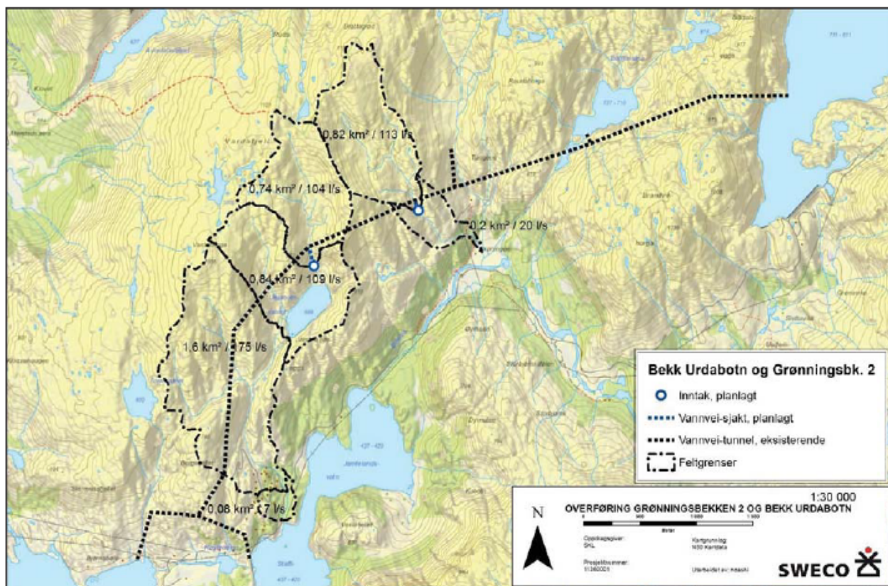
Fig. 2 Planlagt utbygging med inntak i Bekk Urdabotn og i Grøningsbekken 2, høvesvis på kote 720 og 730.
