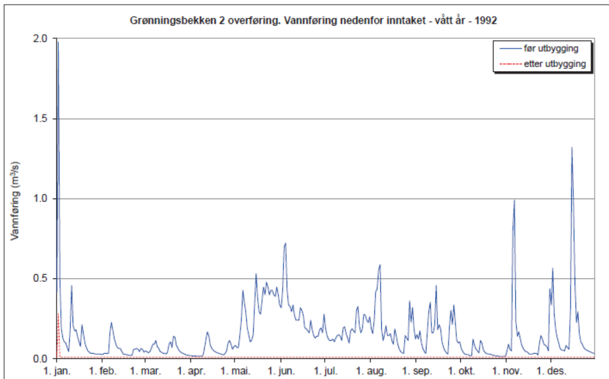
Fig. 5 Vassføring i Grønningsbekken 2 – før og etter utbygging, vått år 1992. Tiltaket vil redusera vassføringa sterkt nedstraums bekkeinntaket, 800 m like til samløp med Blåelva. Det er forslag om slepp av minstevassføring på 10 l/s heile året. Middelvassføringa er i dag 113 l/s.
