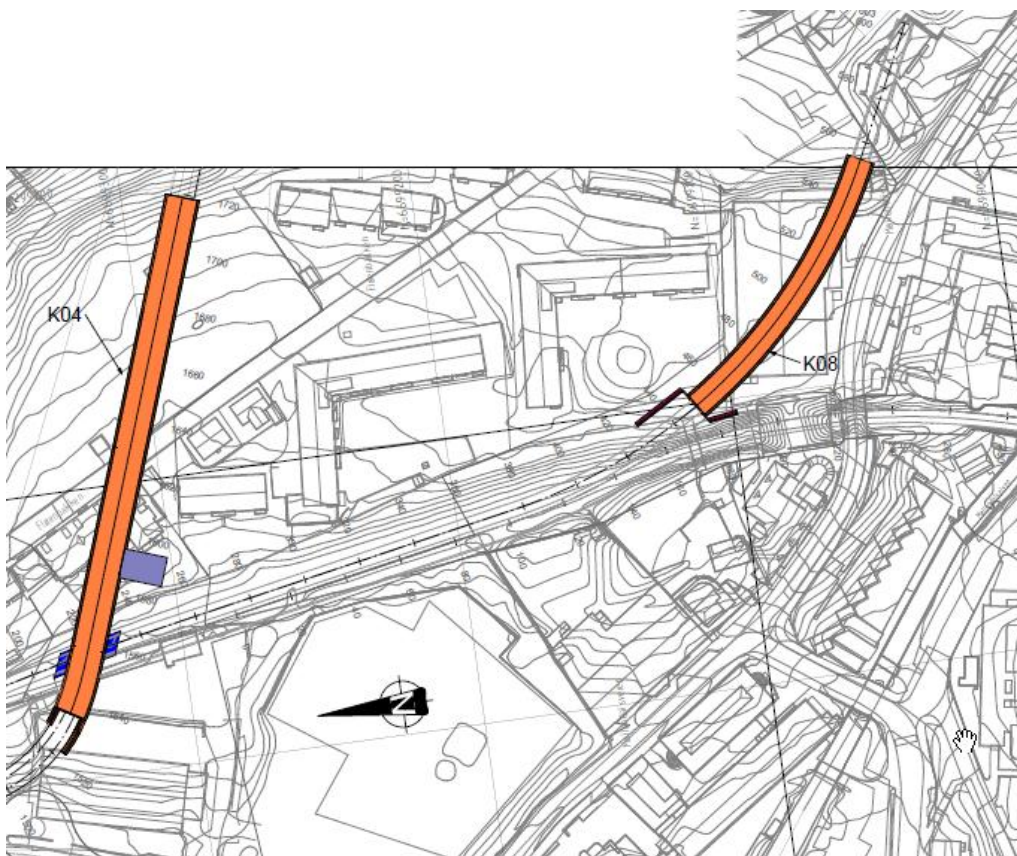
Figur 1: Kartutsnitt med betongportal til uttrekkstunnel til høyre. Stiplet linje over portal viser spor i bergtunnel.
