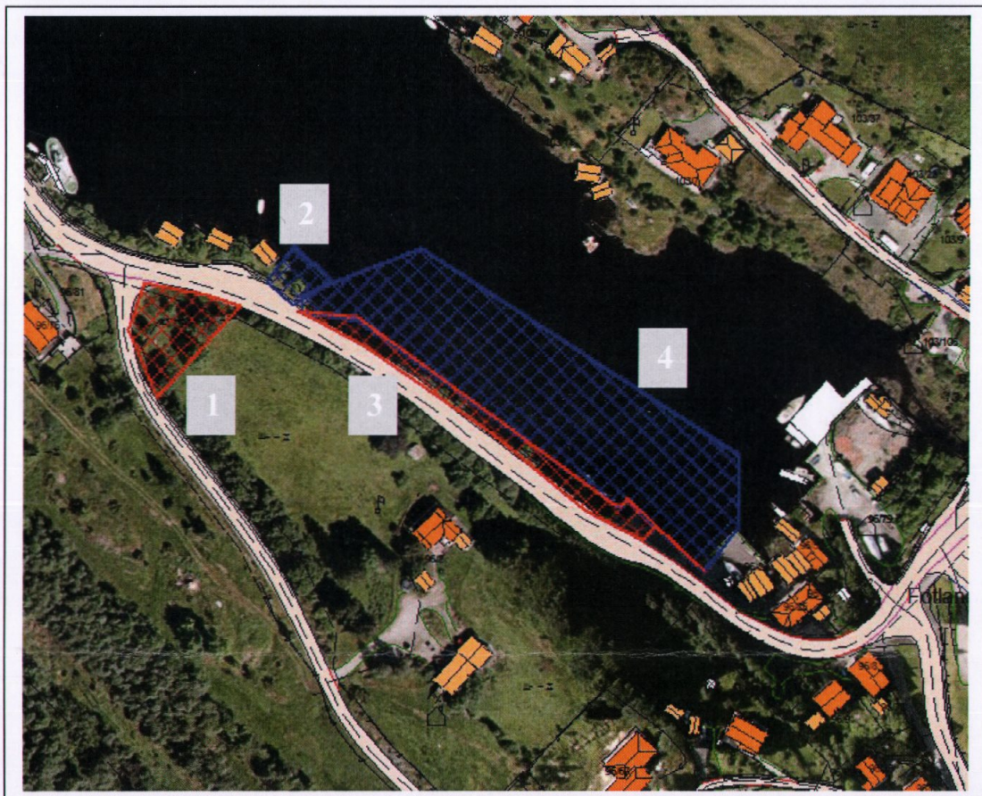
Figur 1. Syner antatt arealbruk ved småbåthamn i Fotlandsvåg (alt. 1). 1) Parkeringsplass, 2) Kai for passasjerbåt, 3) gangveg på flyteelement langs sjø og 4) område for småbåthamn/gjestehamn.
