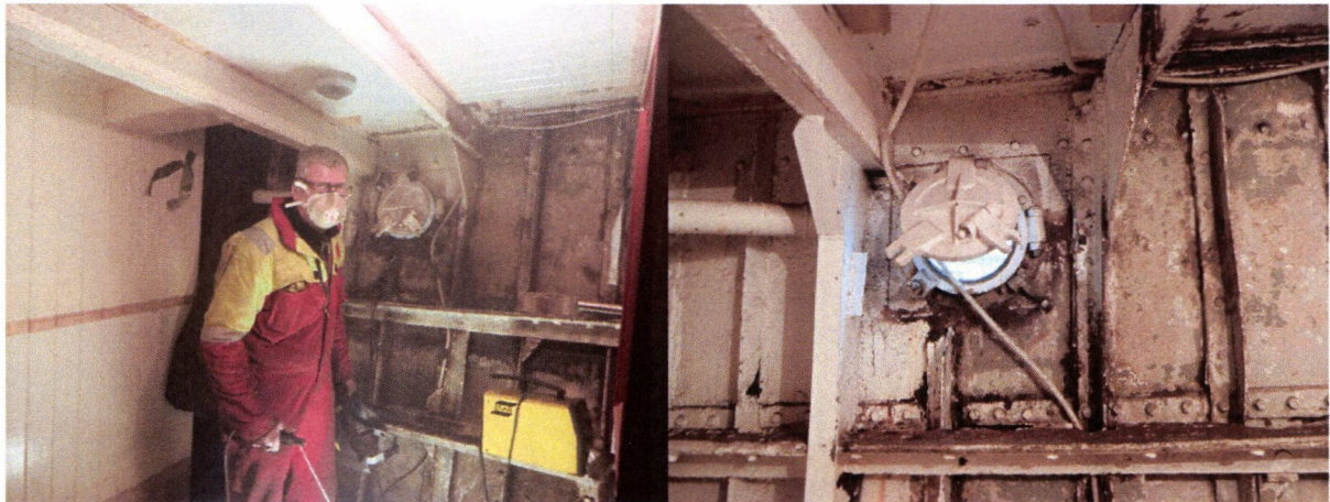
Reparasjon av stål i skuteside i lugarar BB side forskip.
