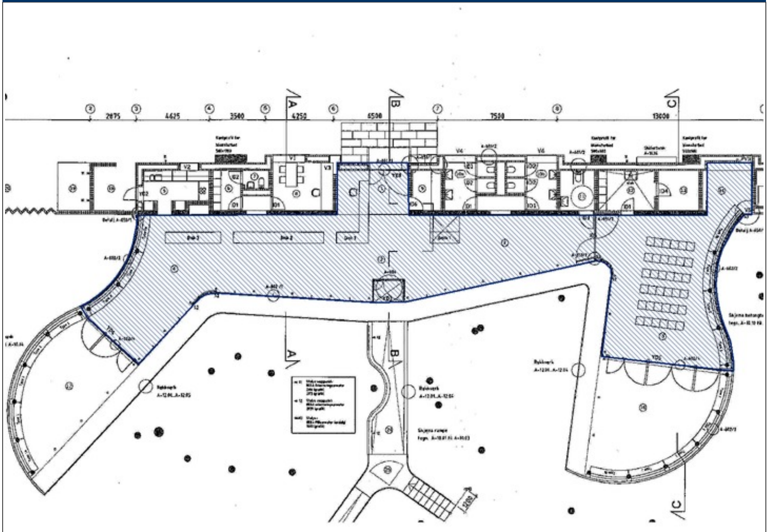
Plantegningen for publikumsbygget. Omfang for interiørfredningen er markert med blå skravur. Gangbanen langs fasaden er ikke utført.
