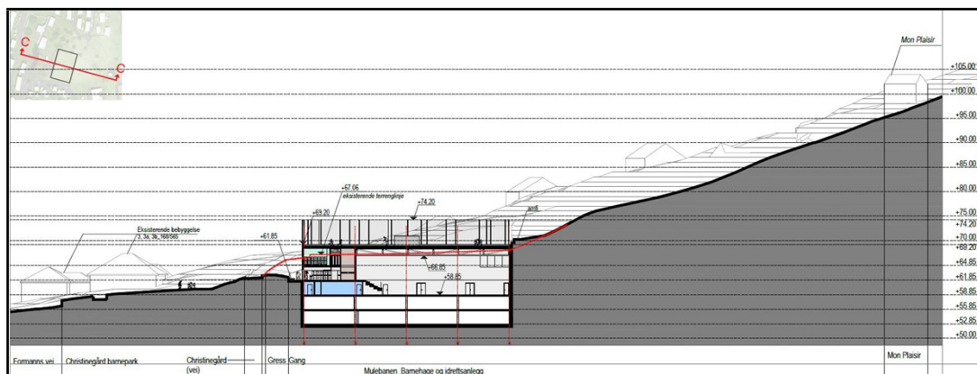
Figur 5 Snitt gjennom fleirbrukshallen sett frå syd
