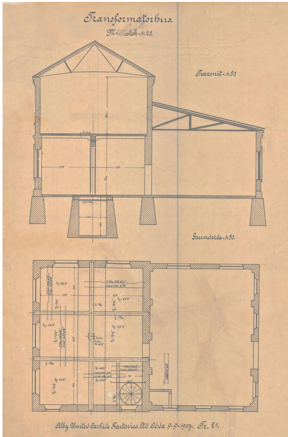
004-Tr.21.Fordelingsstasjon karbid. Alby. 1907 – den fyrste kjende teikninga av Trafostasjonen
