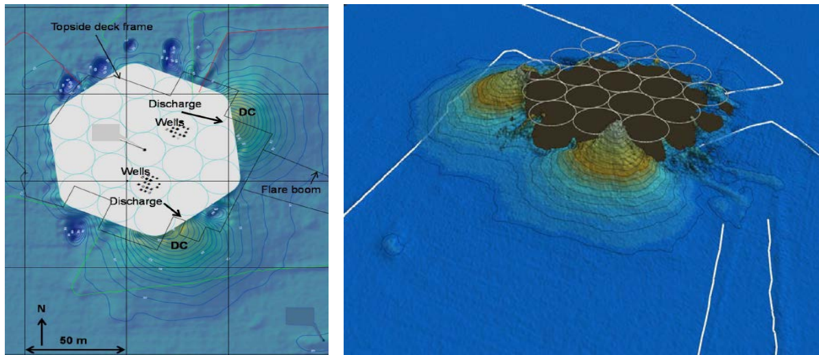
Figur 2-14 Havbunnstopografi rundt SFA. Blå sirkler indikerer lagerceller. Borekaks er markert med DC (DNV, 2012a)
