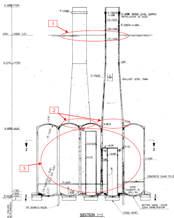
Figur 2-8 Mulige feilscenarier for kollaps av SFA betongunderstell
