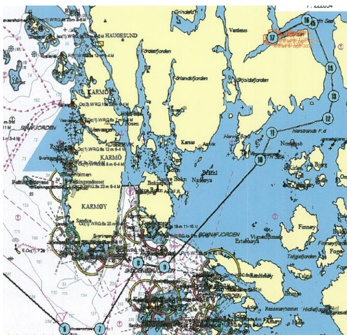
Figur 2-4. Detaljert sleperute for innaskjærs slep fram til oppankringslokalitet i Yrkefjorden.
